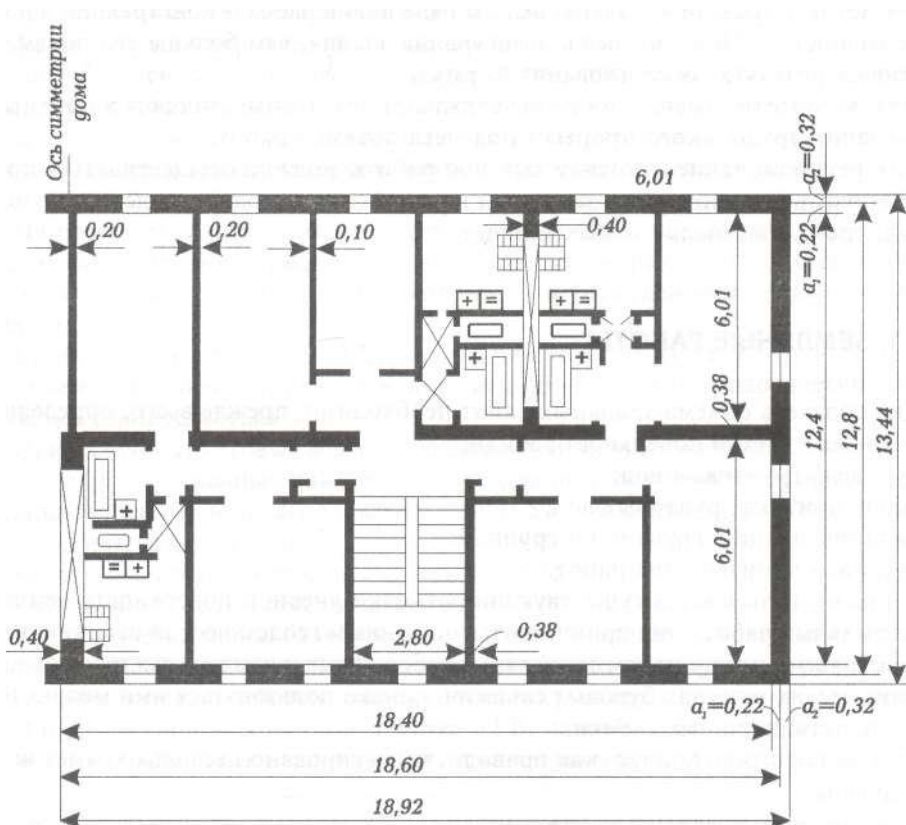
Рис. 6. План типового этажа
