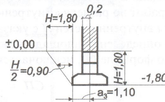
Рис. 5. Сечение по наружным фундаментам и котловану
