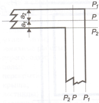
Рис. 2. Угол наружных стен здания
