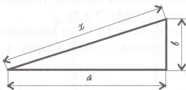
Рис. 4. Схема уклона кровли
