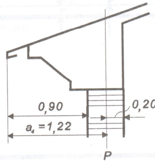
Рис. 3. Сечение по свесу кровли
